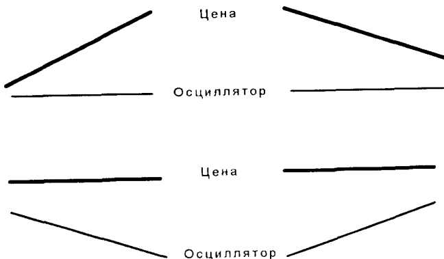
Рис. 7—5. Три типа дивергенции
