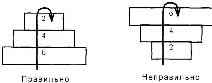
Рис. 9—12. Правило построения пирамиды при добавлении позиций
